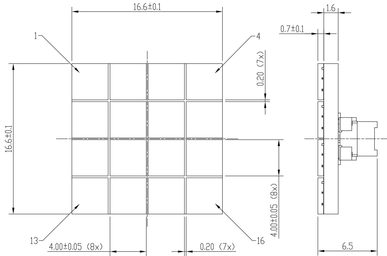
Top View Scale: 5 : 1
